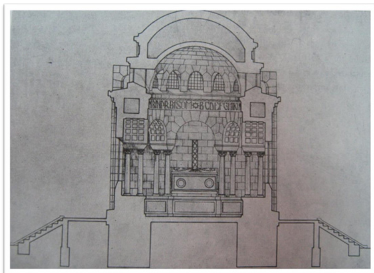
Secțiune – desen, proiectul arhitectului Duiliu Marcu
